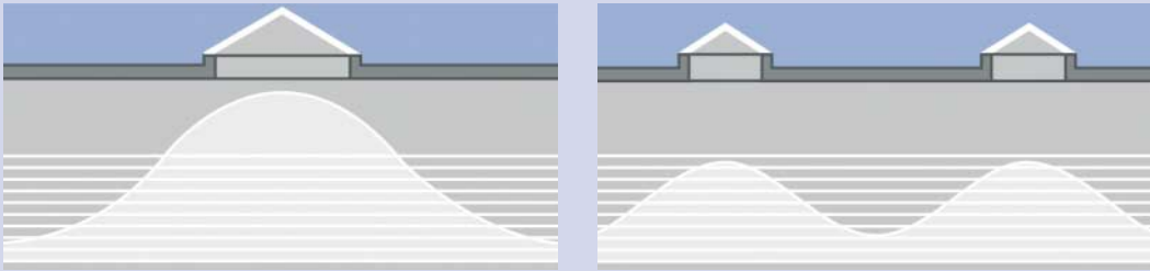
Bild 11: Anordnung, Größe und Anzahl der Dachoberlichter bestimmen die Verteilung des Tageslichts im Raum.
